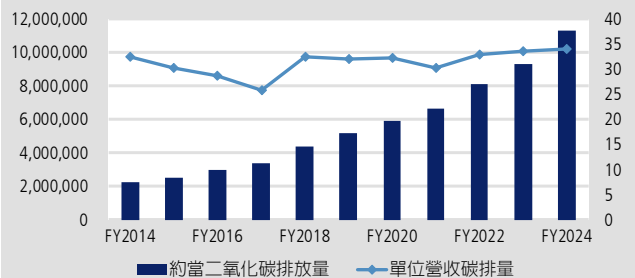
圖 18：Alphabet – 碳排放量
